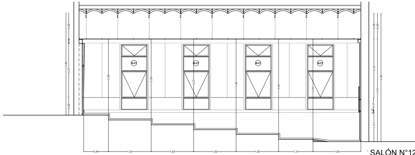
SALÓN N°12 CORTE AA
