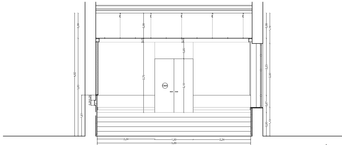
SALÓN N°12 CORTE BB
