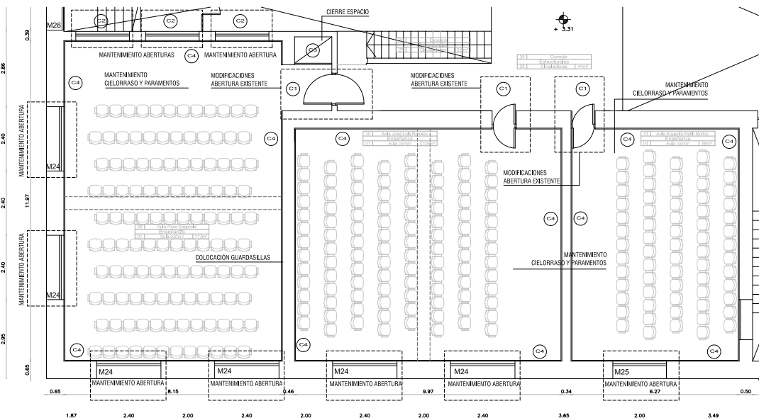
PLANTA ALBAÑILERÍA SECTOR SALONES ESC. 1/200
